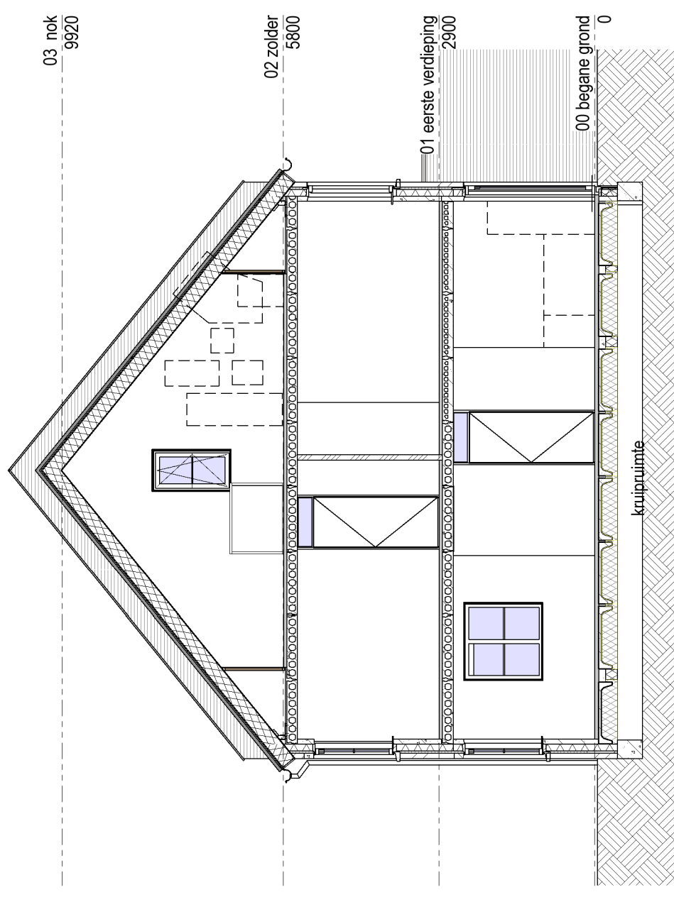
doorsnede bouwnummer 143
