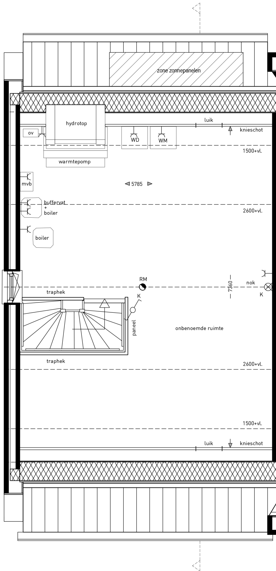
bouwnr 143
