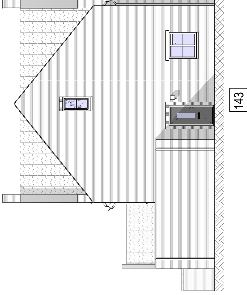
linker zijgevel
