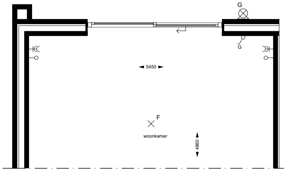
Begane grond schuifpui
