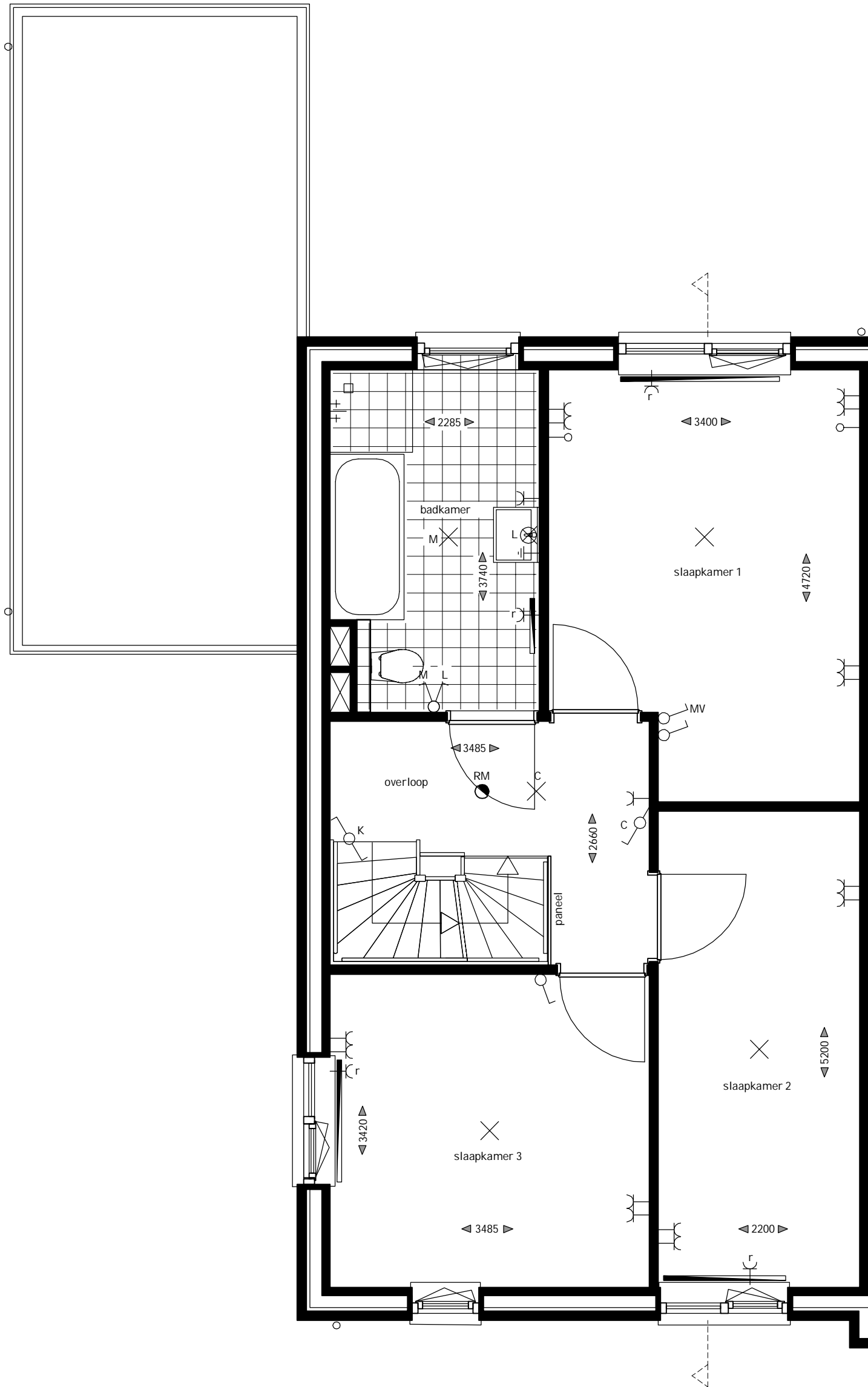
bouwnr 145
