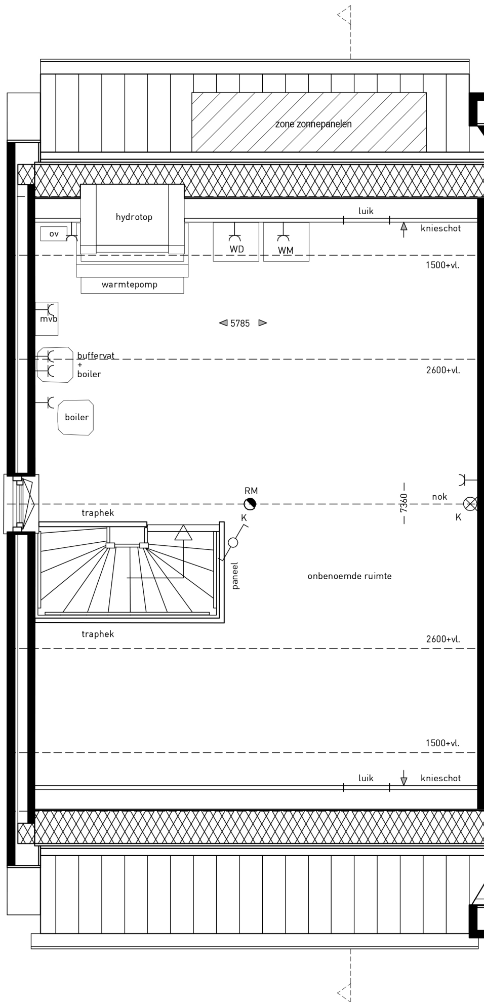
bouwnr 145
