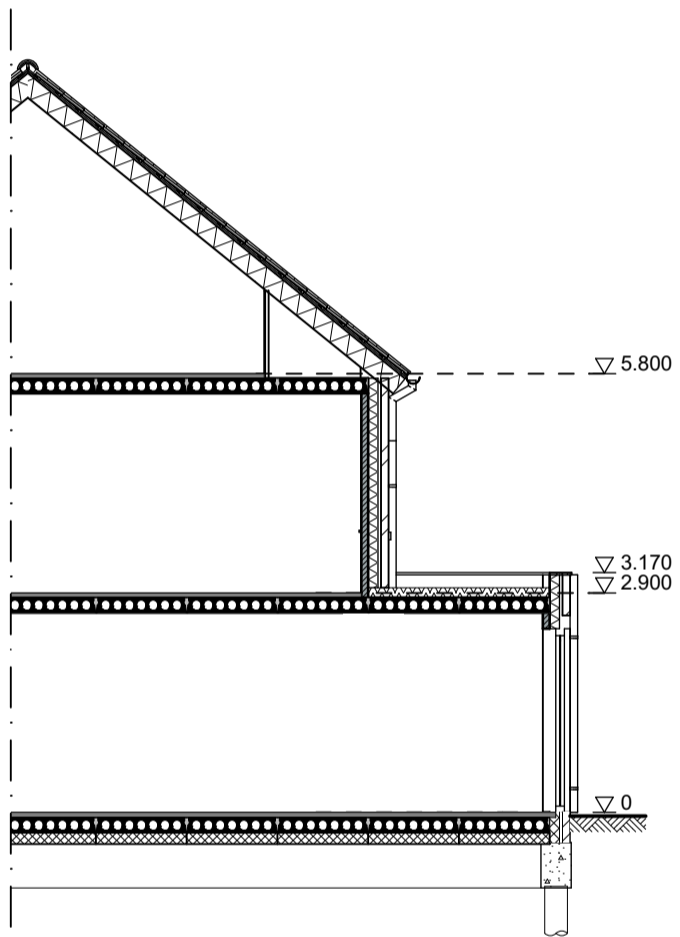
Doorsnede 2400+
