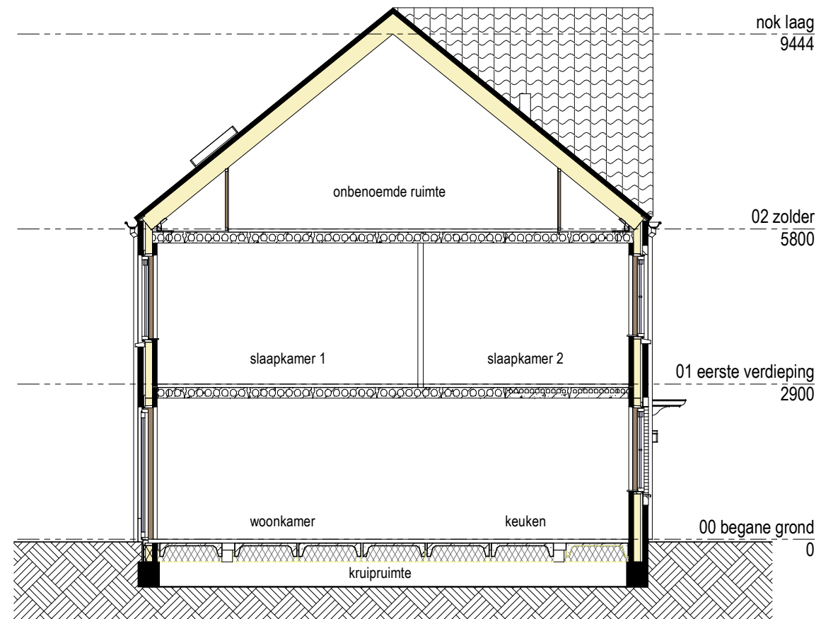
Doorsnede A-A
