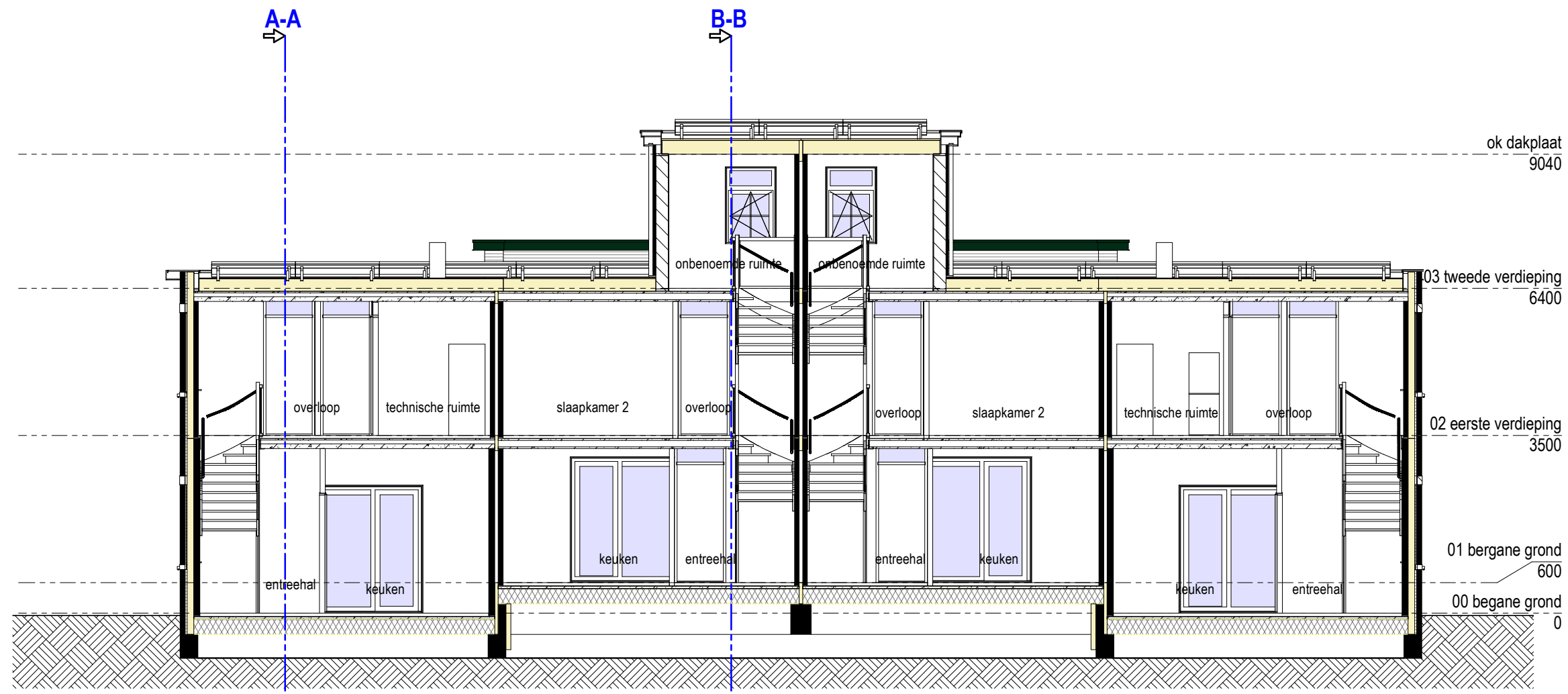
Doorsnede C-C
