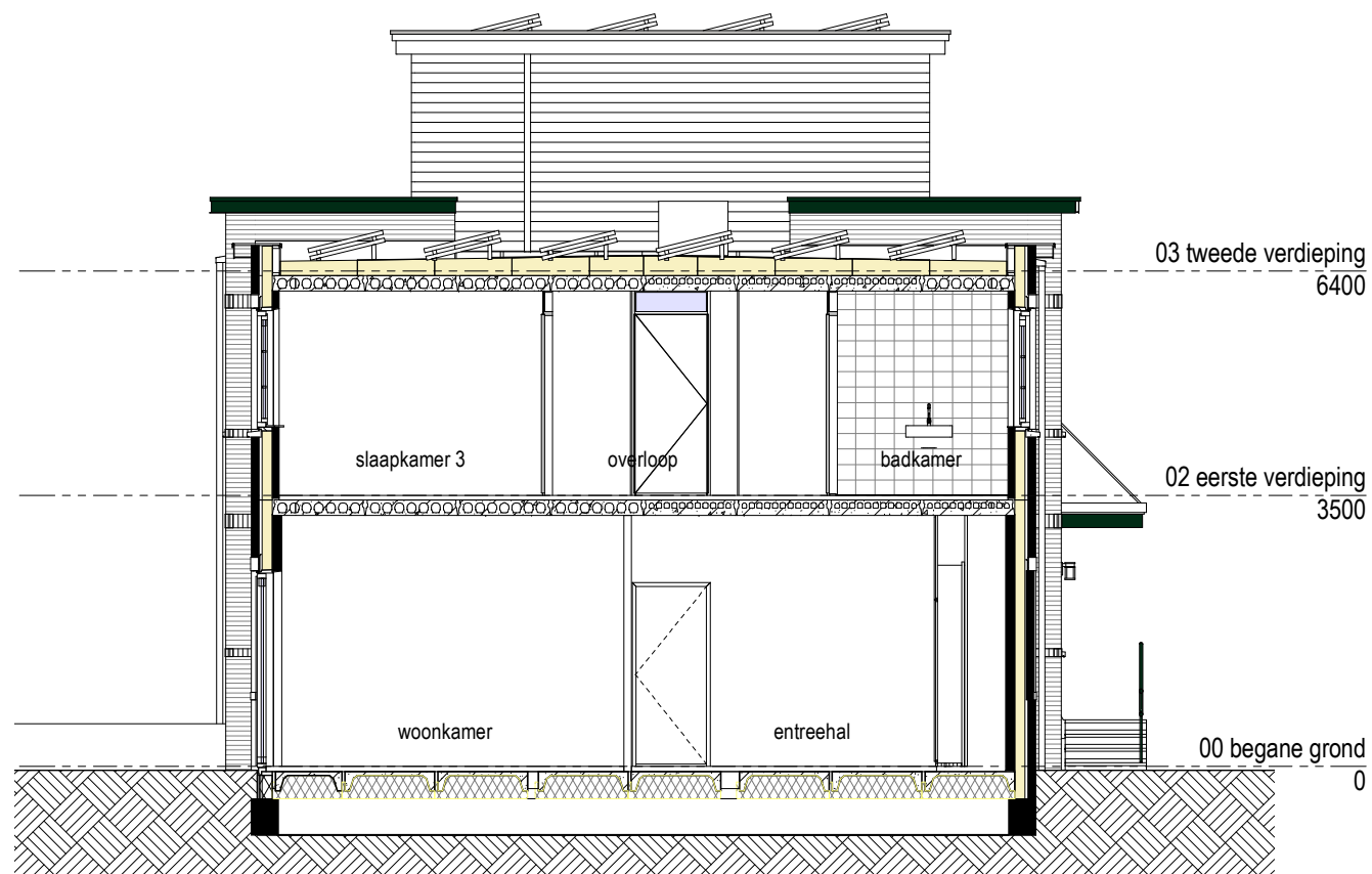
Doorsnede A-A
