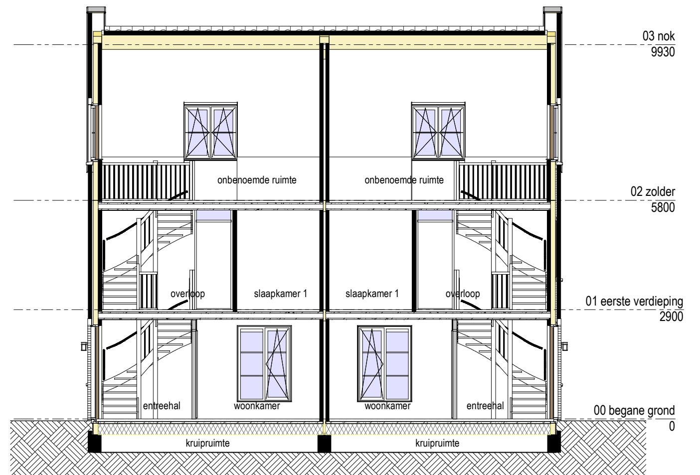
Doorsnede B-B
