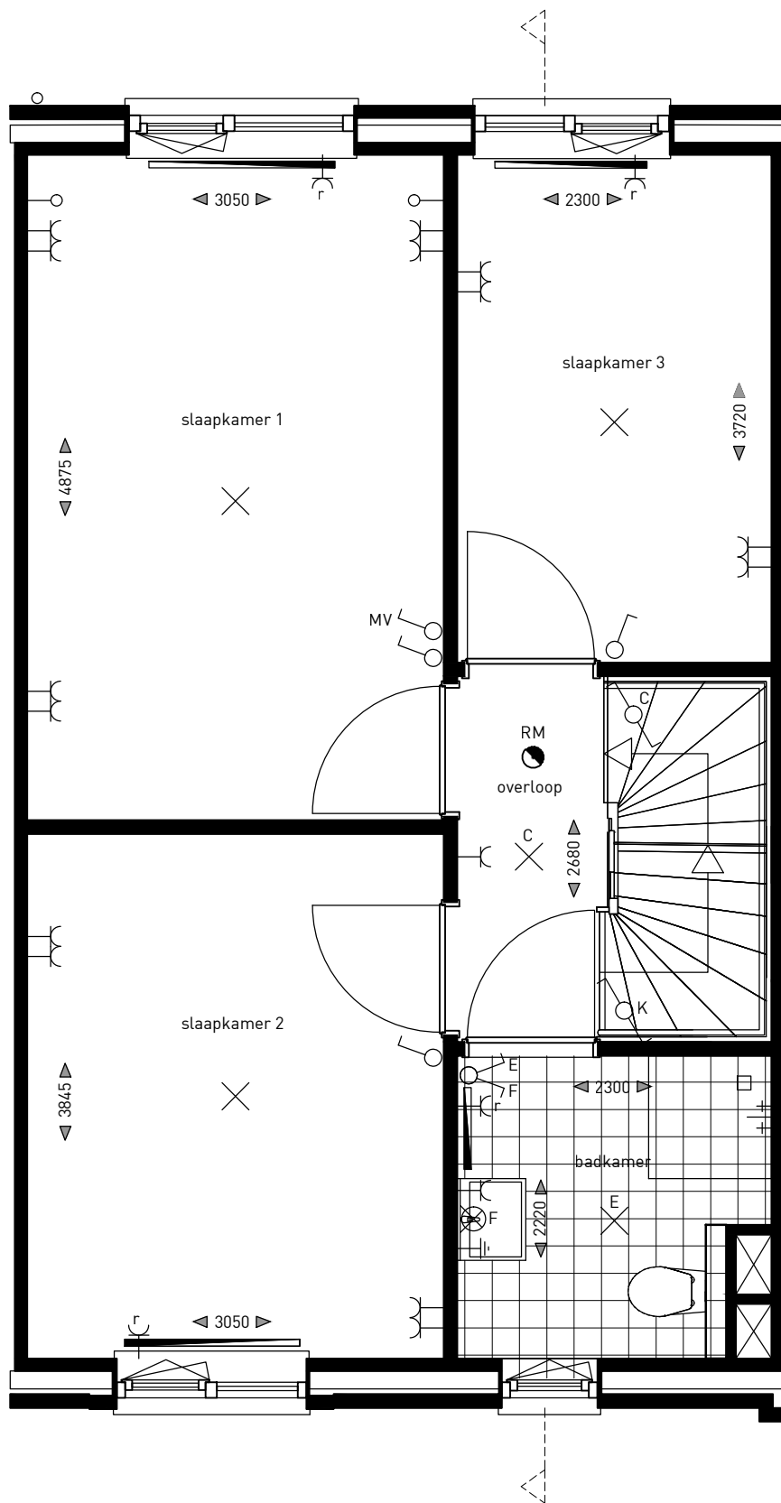
bouwnr 342
