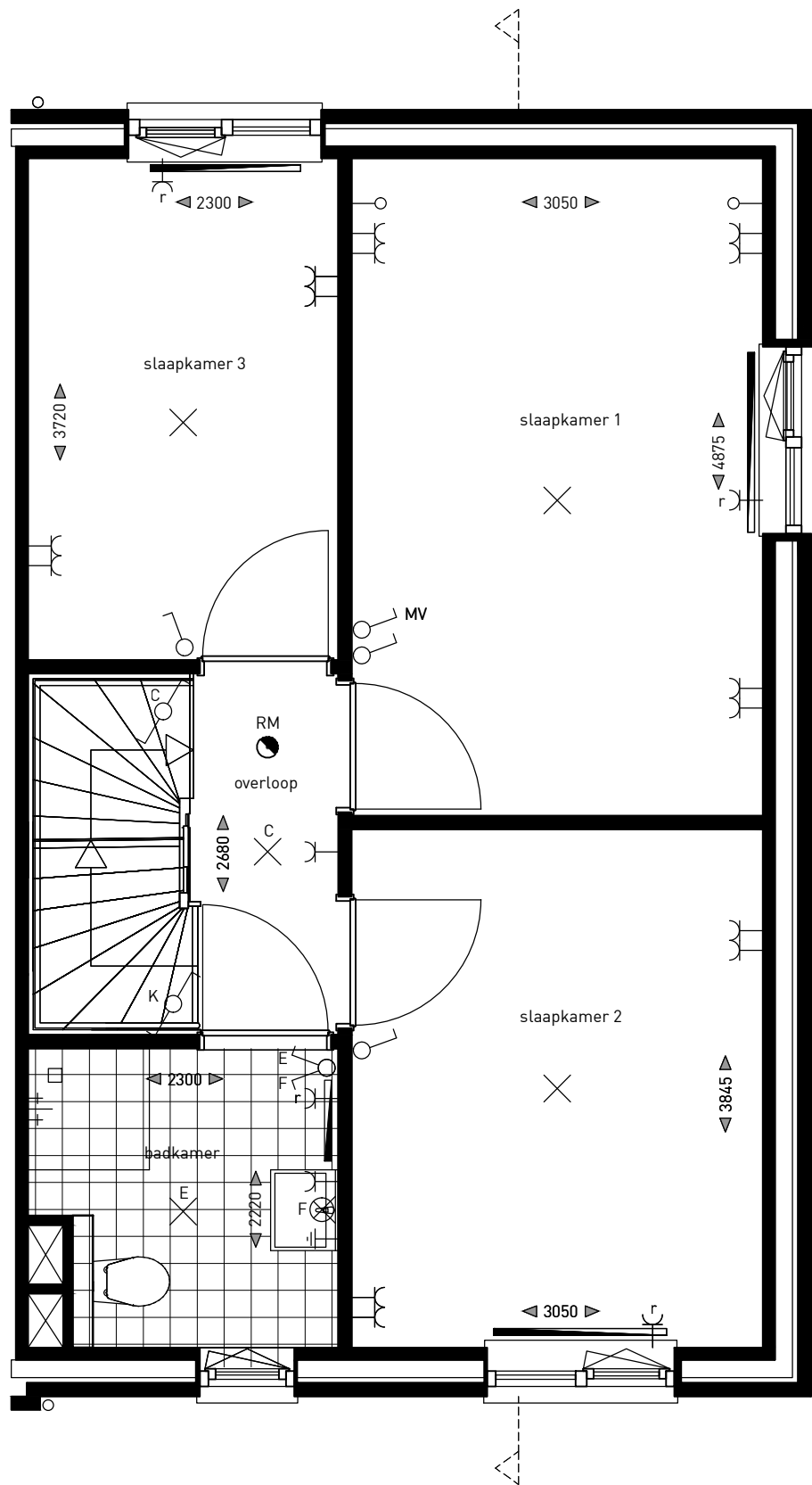
bouwnr 341
