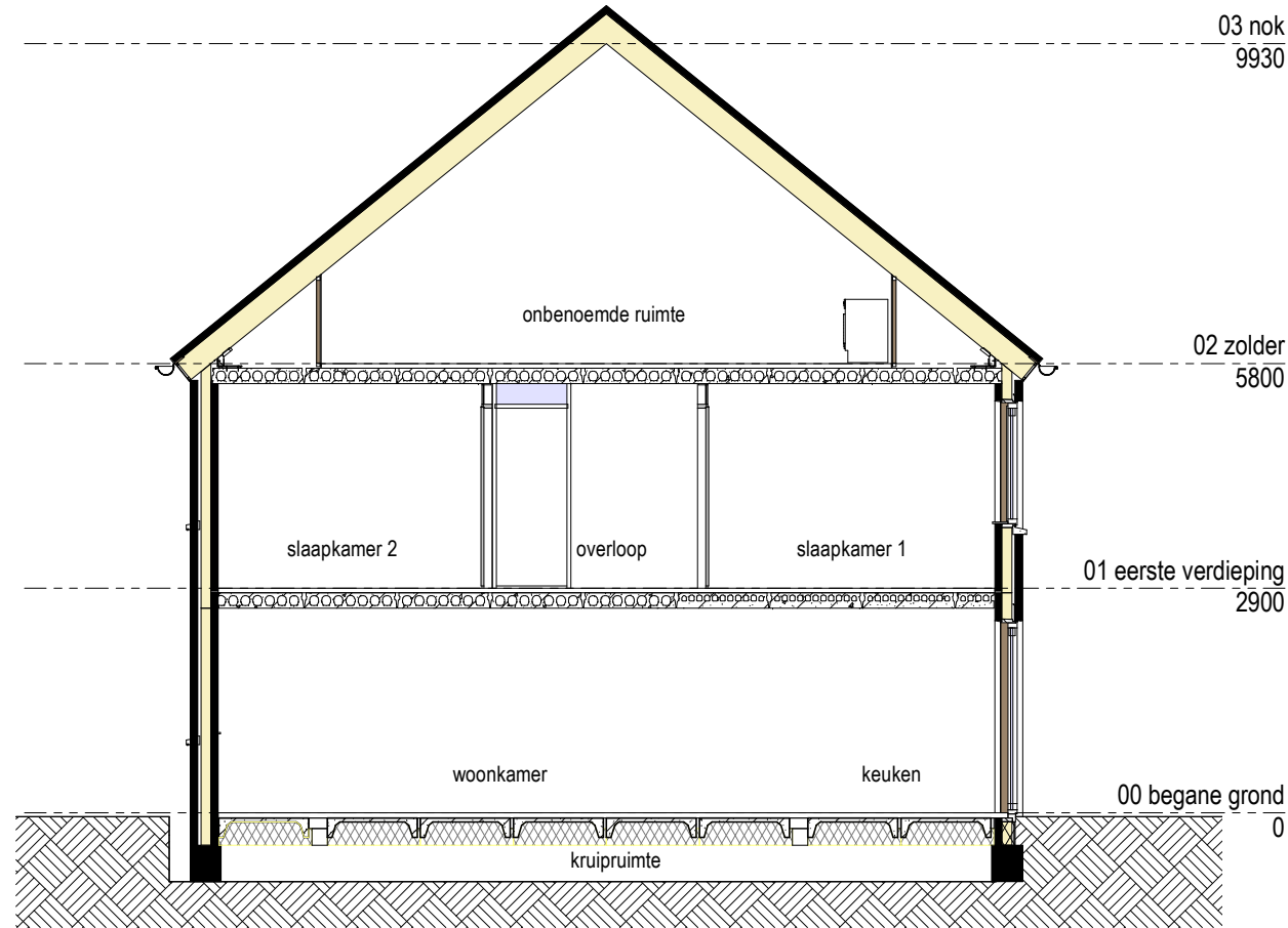
Doorsnede A-A
