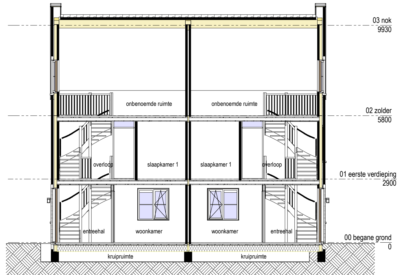
Doorsnede B-B 400
