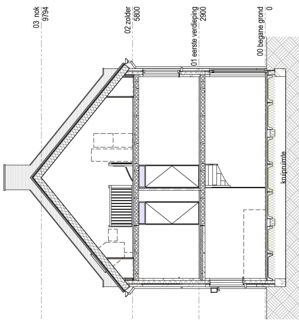
doorsnede bouwnummer 173
