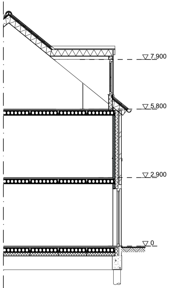
Doorsnede dakkapel
