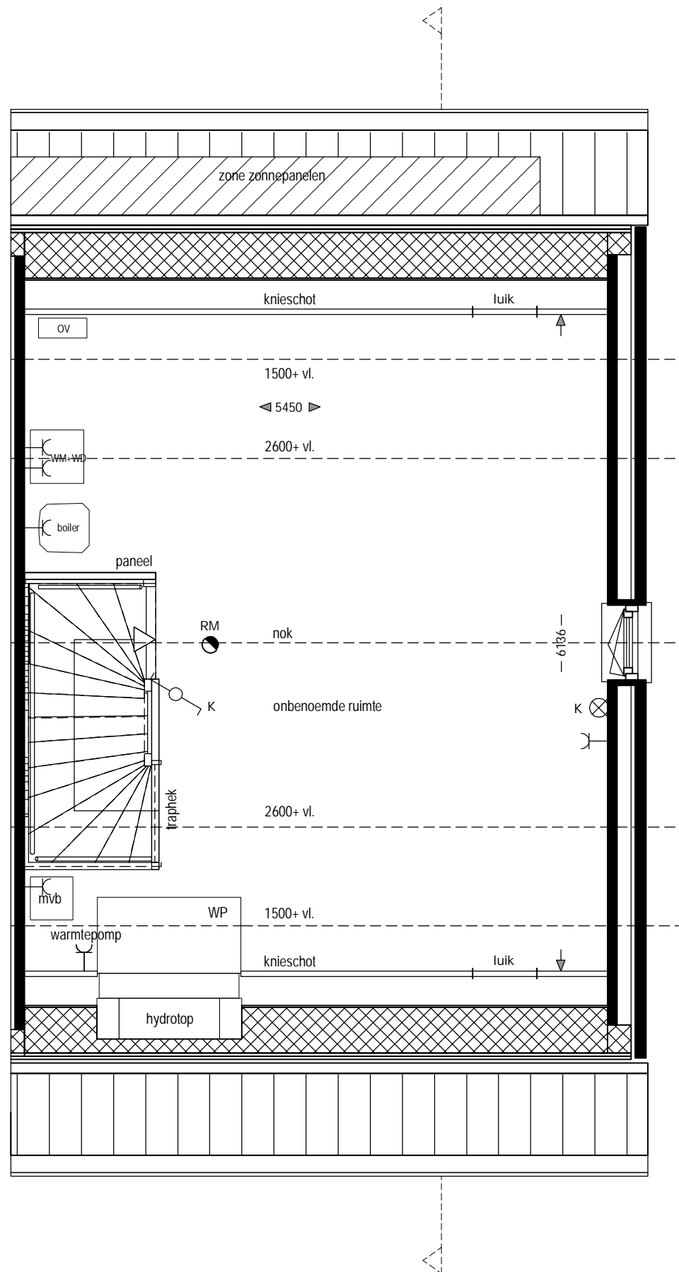
bouwnr 337
