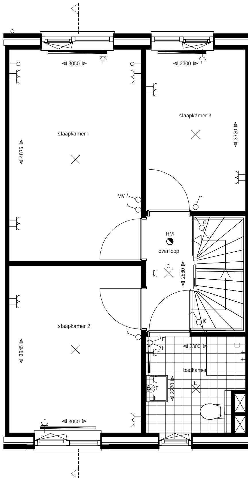
bouwnr 338
