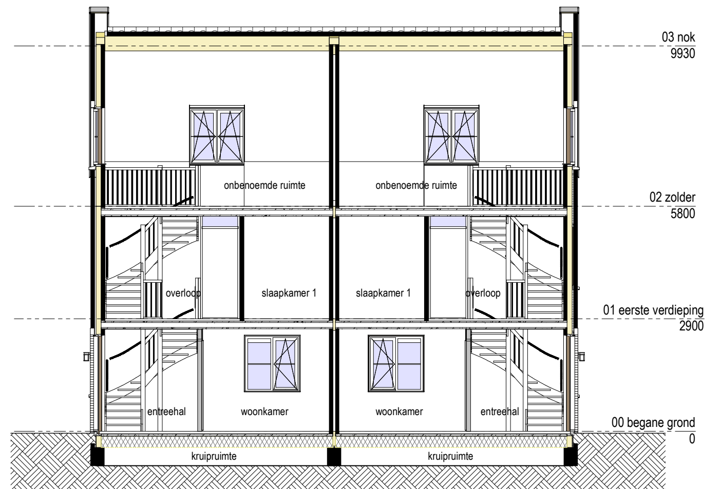
Doorsnede B-B 359
